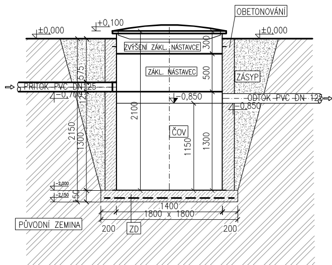
Řez
