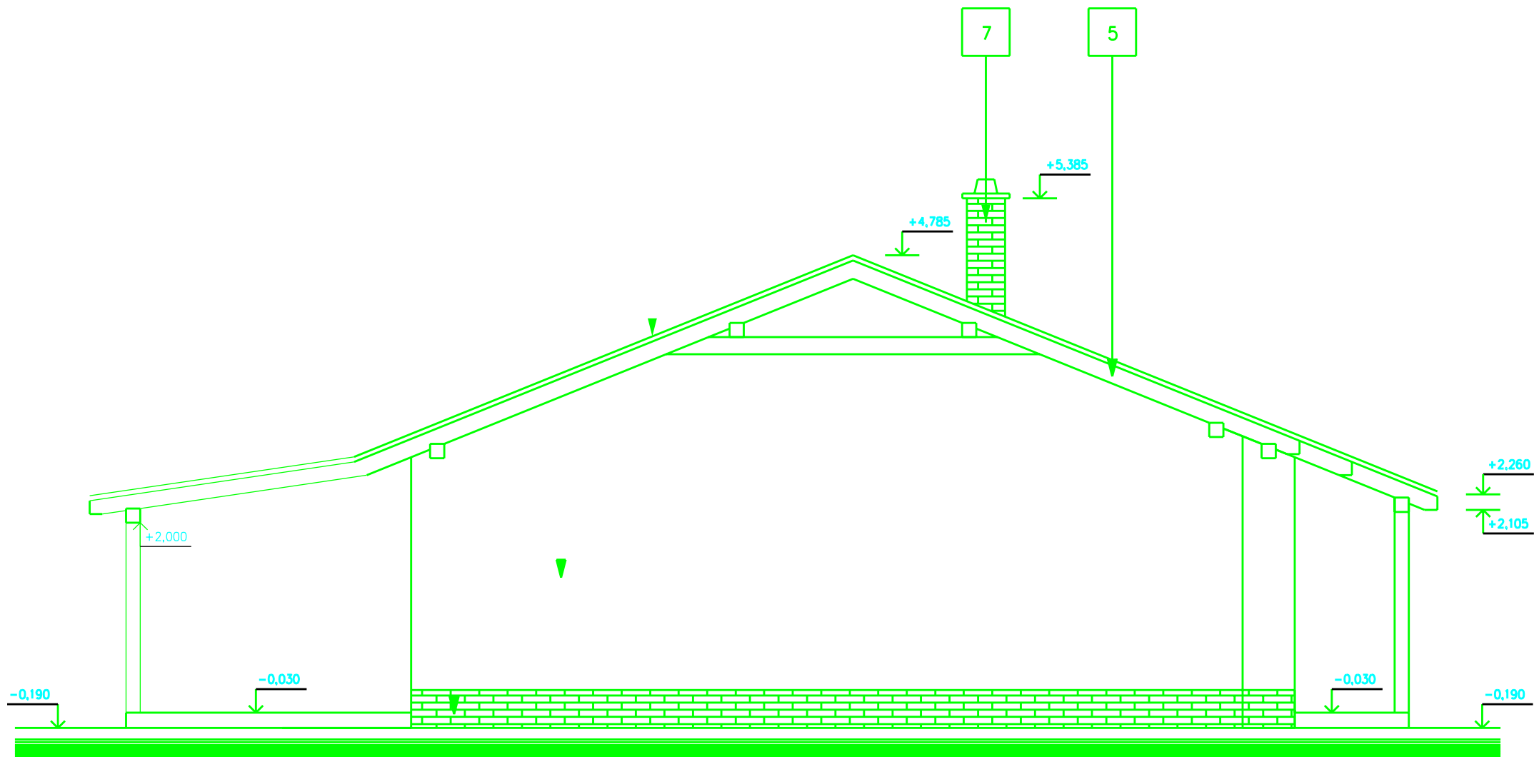
POHLAD BOČNÝ
