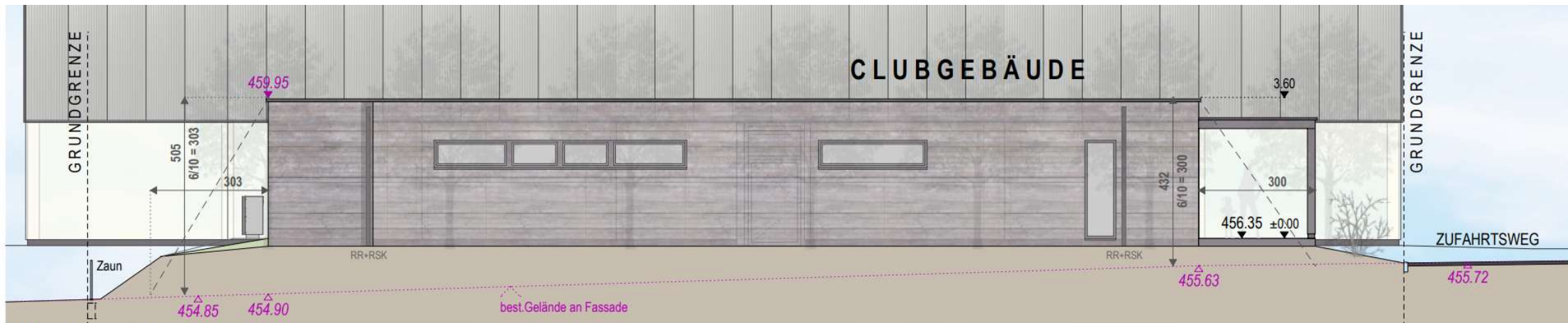
Westansicht M1:100
