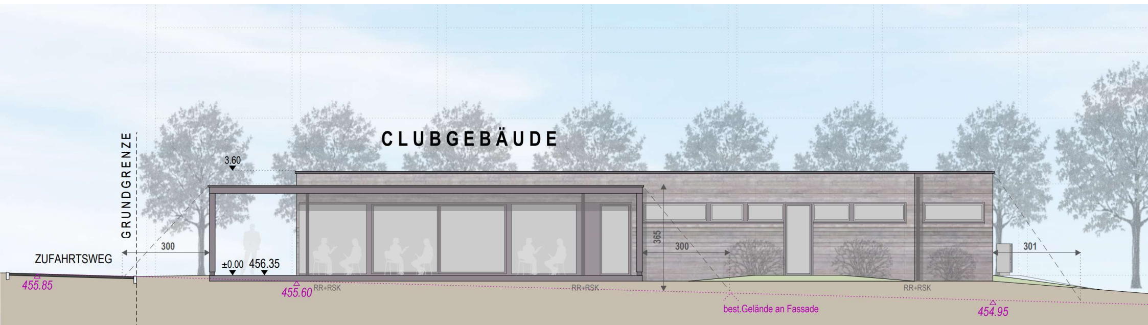
Ostansicht Clubgebäude M1:100
