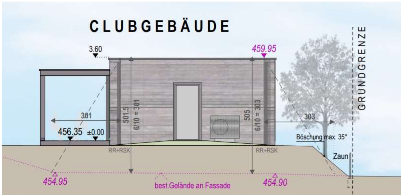
Nordansicht M1:100
