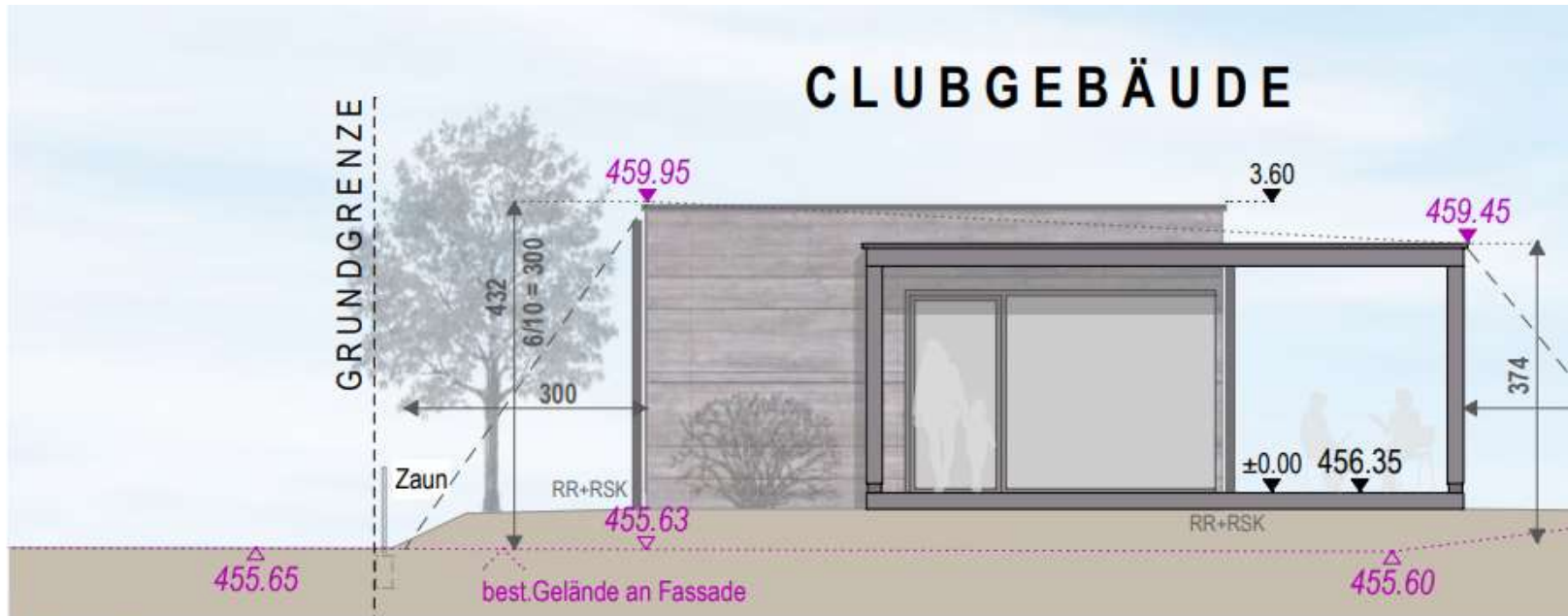
Südansicht M1:100
