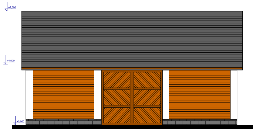
Pohledy severní a jižní 1 : 100
