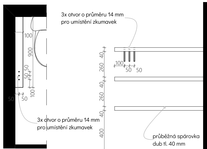
PŮDORYS M 1:20 POHLED M 1:20
