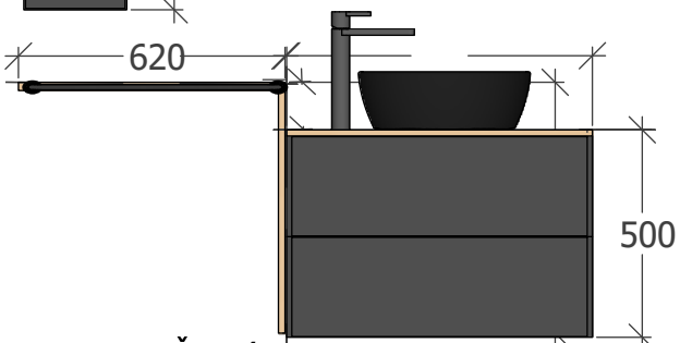
POHLED ČELNÍ
