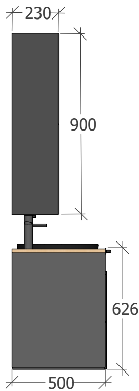
POHLED BOČNÍ
