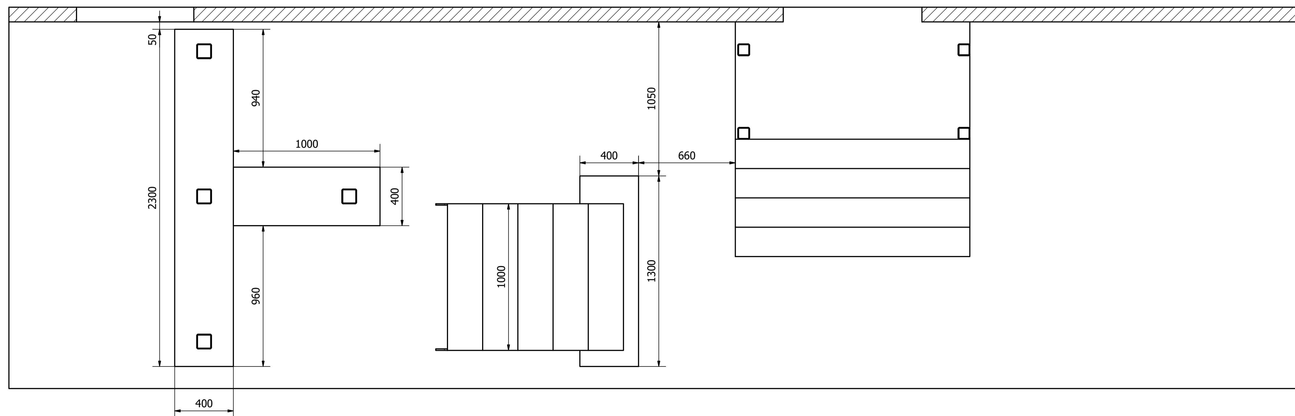
A-A ( 1 : 15 )
