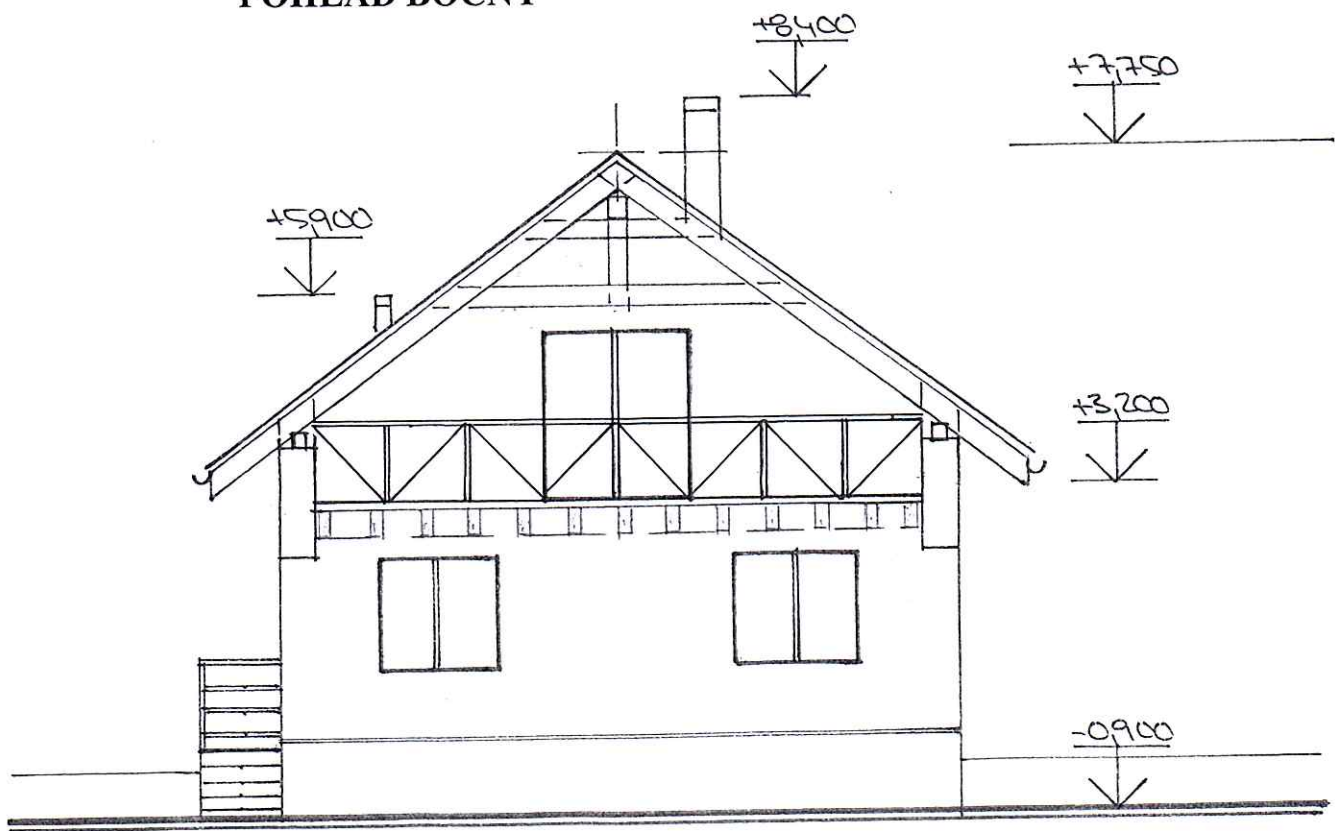
POHLED BOČNÝ
