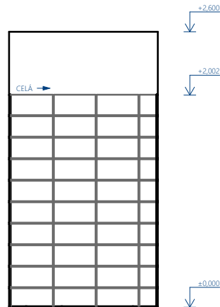
IP-02 1:50
