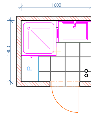
Půdorys sanita 1:50
