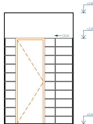
IP-03 1:50
