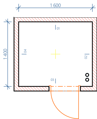
Půdorys 1:50
