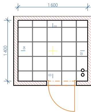
Půdorys spárořez 1:50
