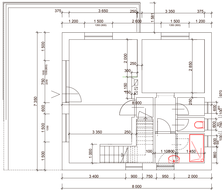
PŘÍZEMÍ návrh
