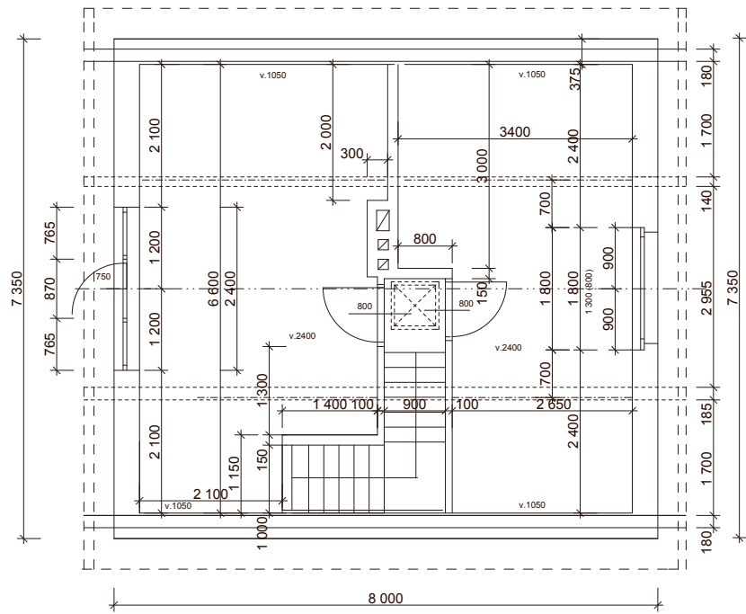
PODKROVÍ stávající stav
