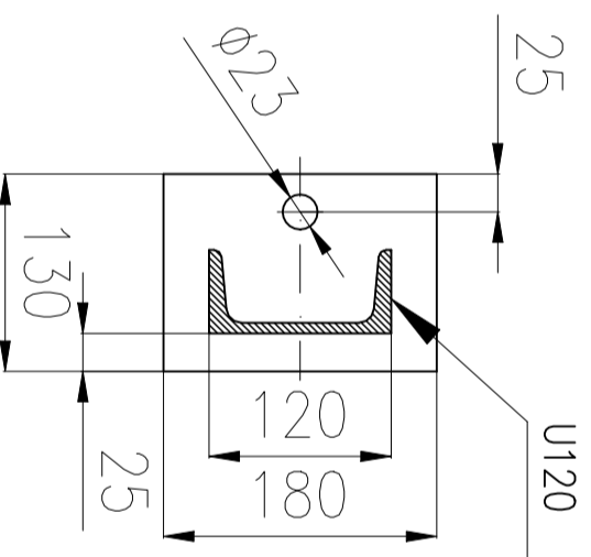
PATKA ŘEZ A-A M2:5
