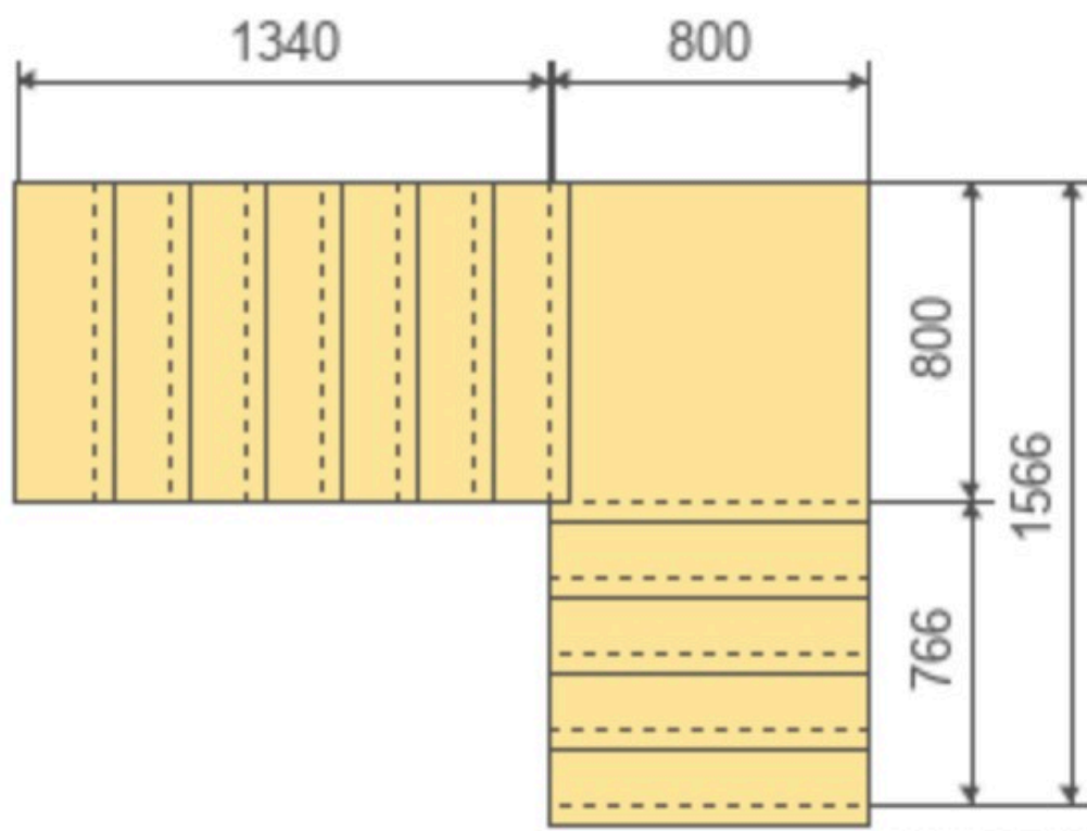
Celý výkres schodiště
