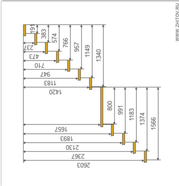
Výkres šablony schodiště
