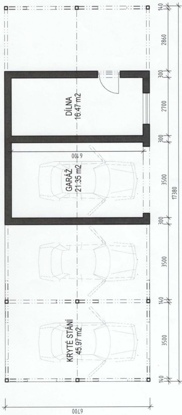
půdorys
