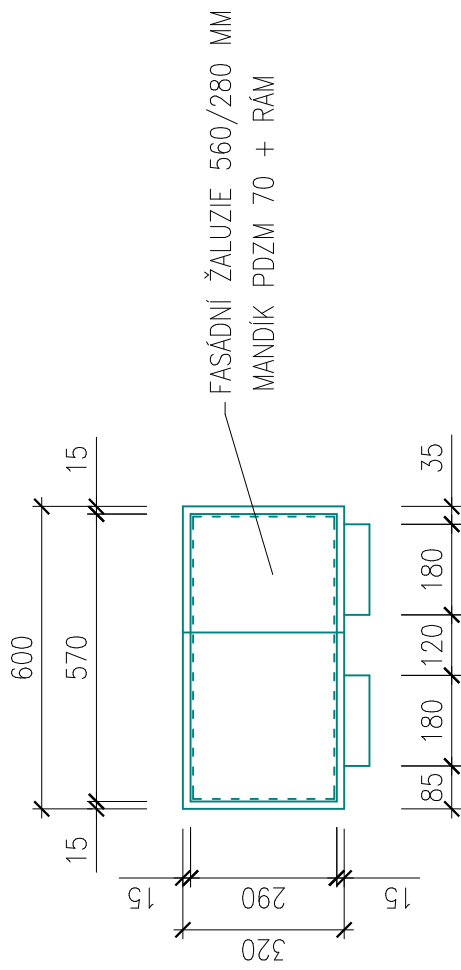
ČELNÍ POHLED
