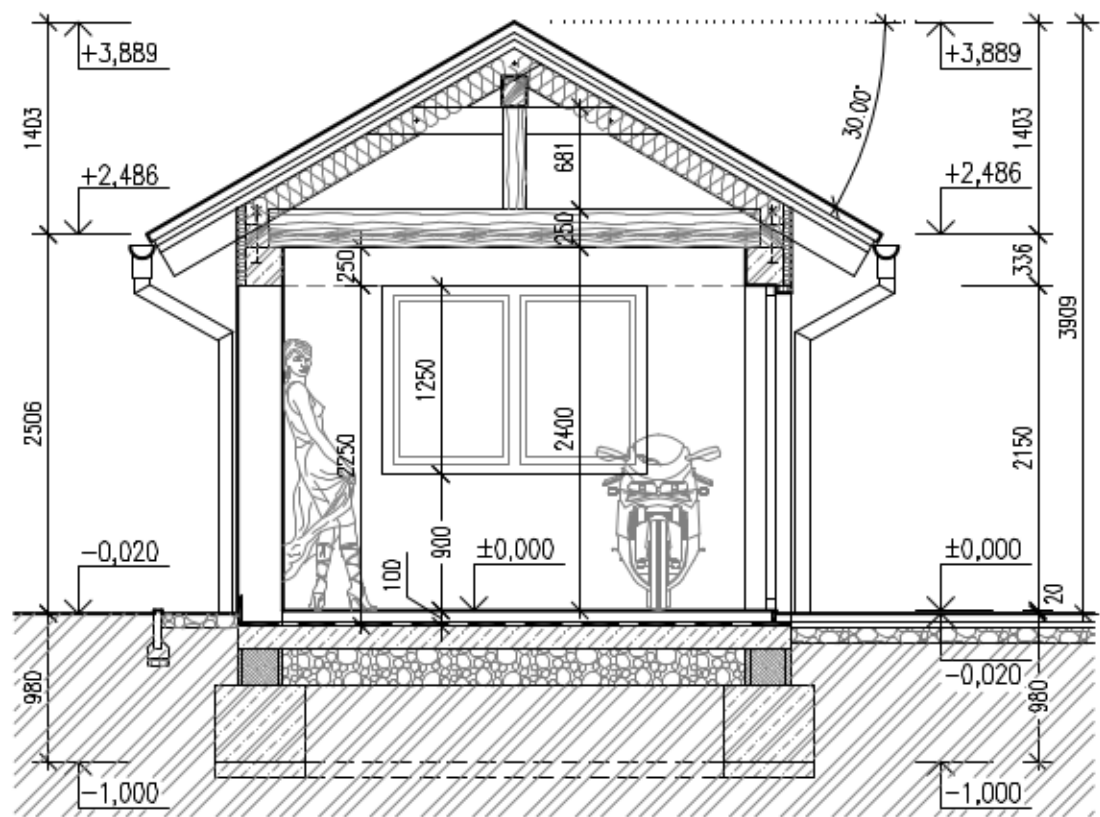
PRIEČNY REZ A-A
