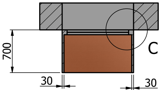
ŘEZ B-B
