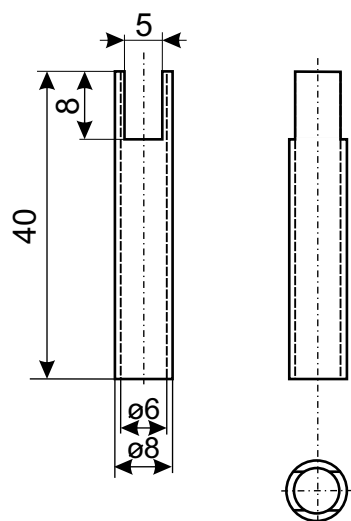
PODPĚRA mat. trubka nerez prům.8/6 mm M1:1
