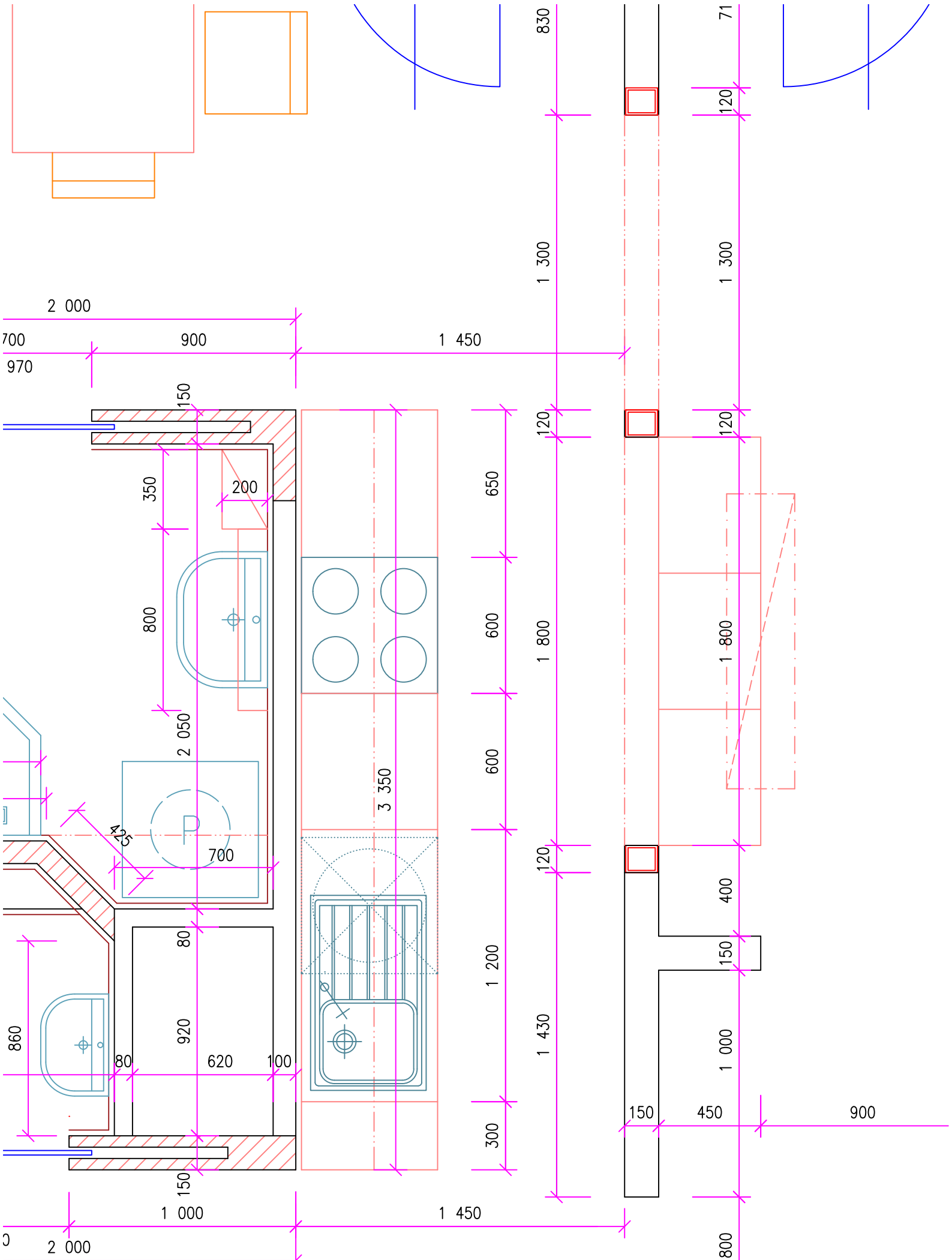
KUCHYŇ ÚSTÍ - PŮDORYS v_1 - M 1 : 20
