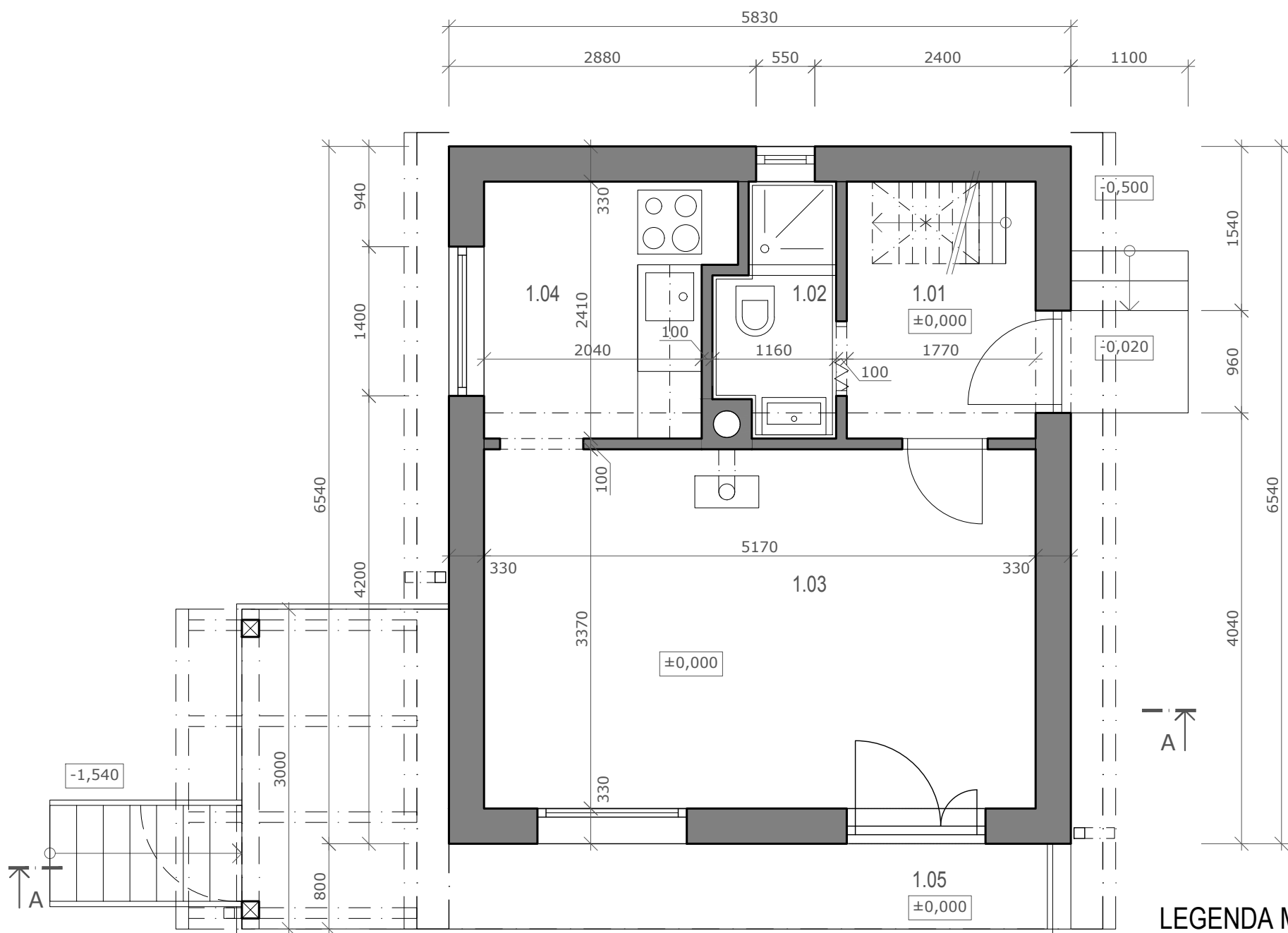
PÔDORYS 1.NP, m1:50
