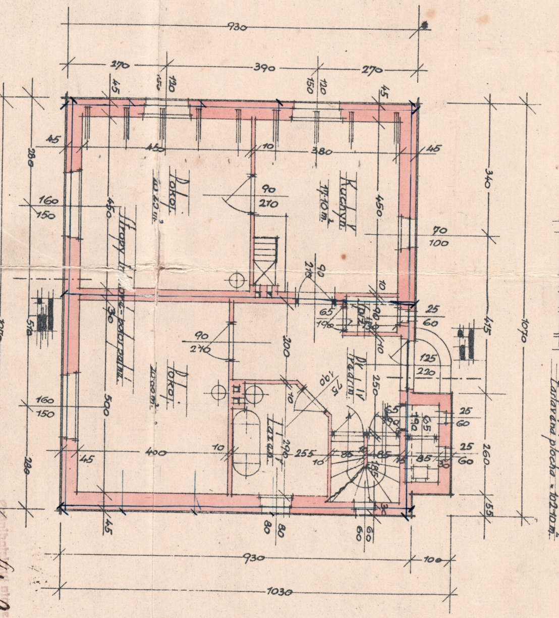
PRÍZEMÍ
