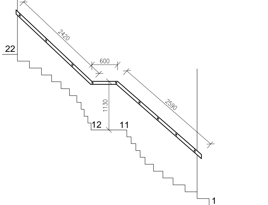
ROZVINUTÝ POHLED / 1:50
