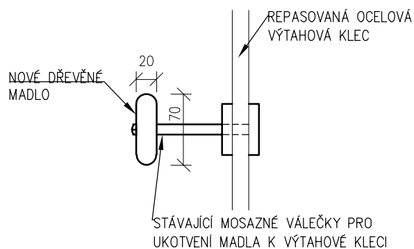
ŘEZ MADLEM 1:5
