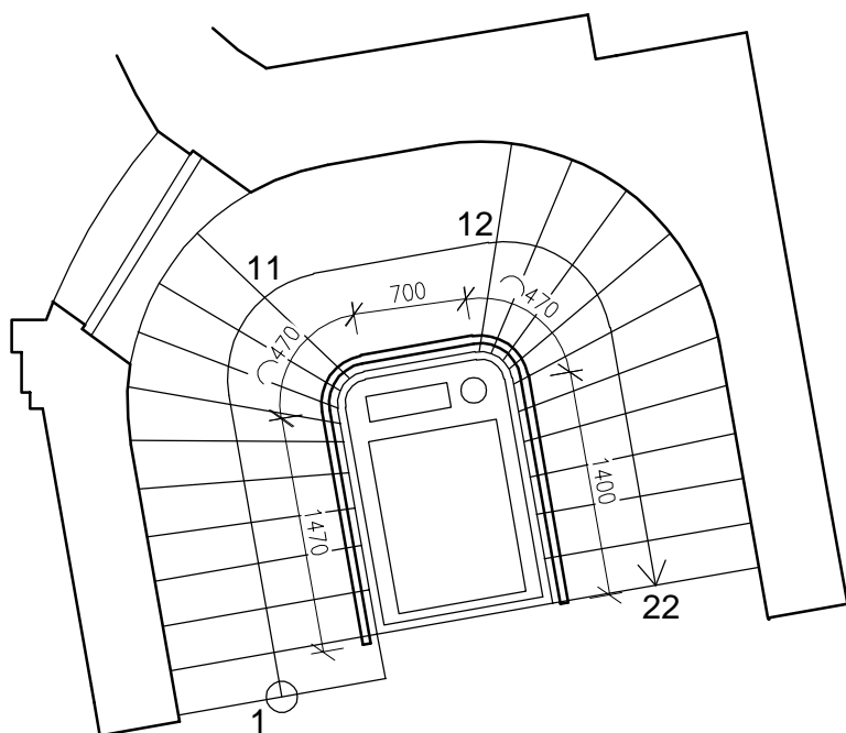
PŮDORYS / 1:50
