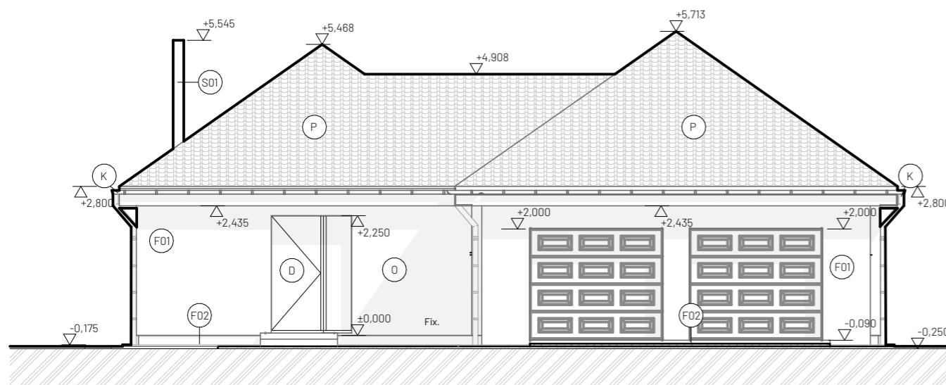
Pohled severní
