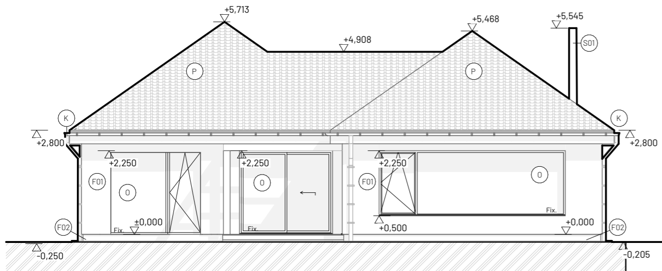
Pohled jižní
