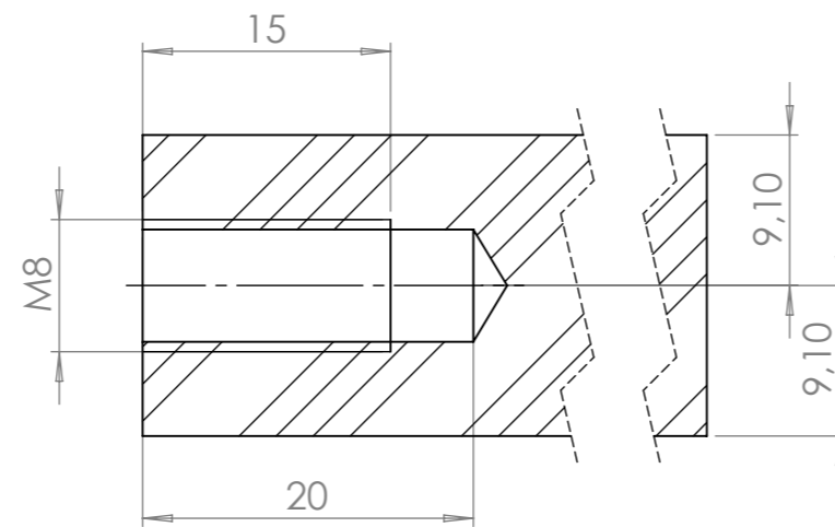
ŘEZ A-A
