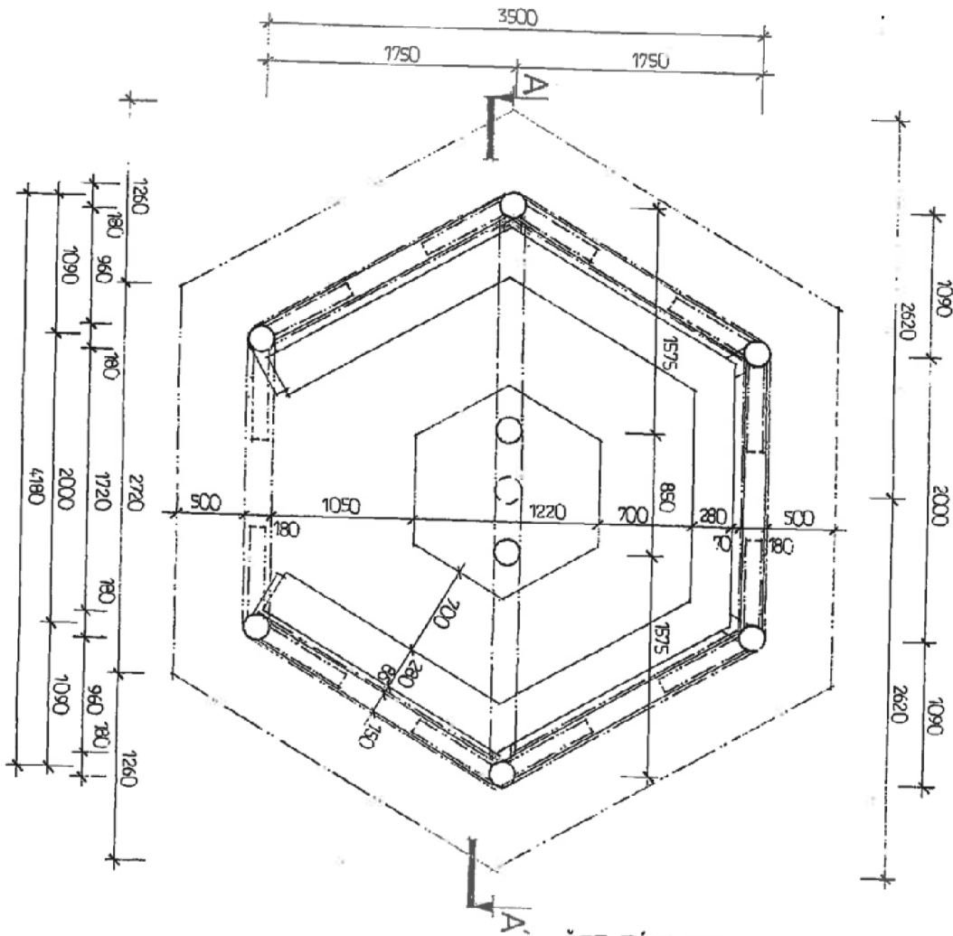
PŮDORYS KROVU M 1:40
