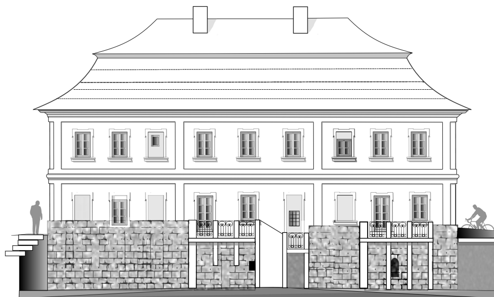
POHLED OD VÝCHODU
