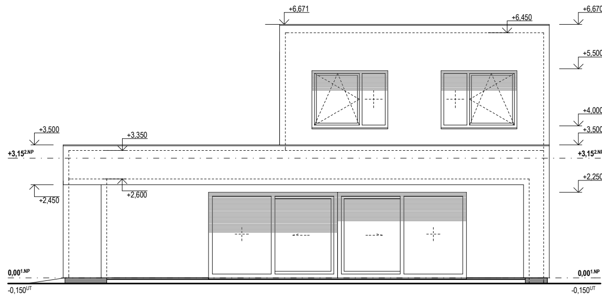
JZ POHLED
