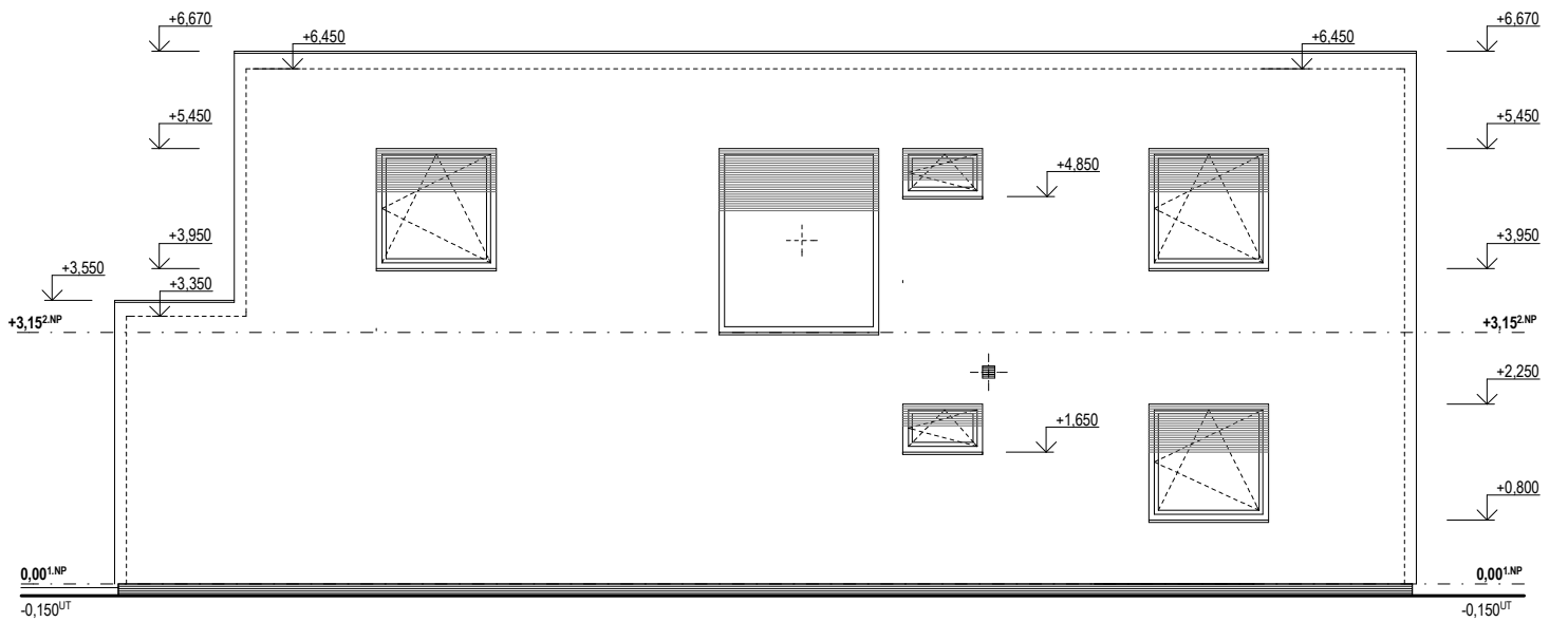
JV POHLED
