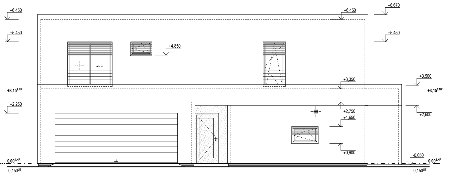
SZ POHLED
