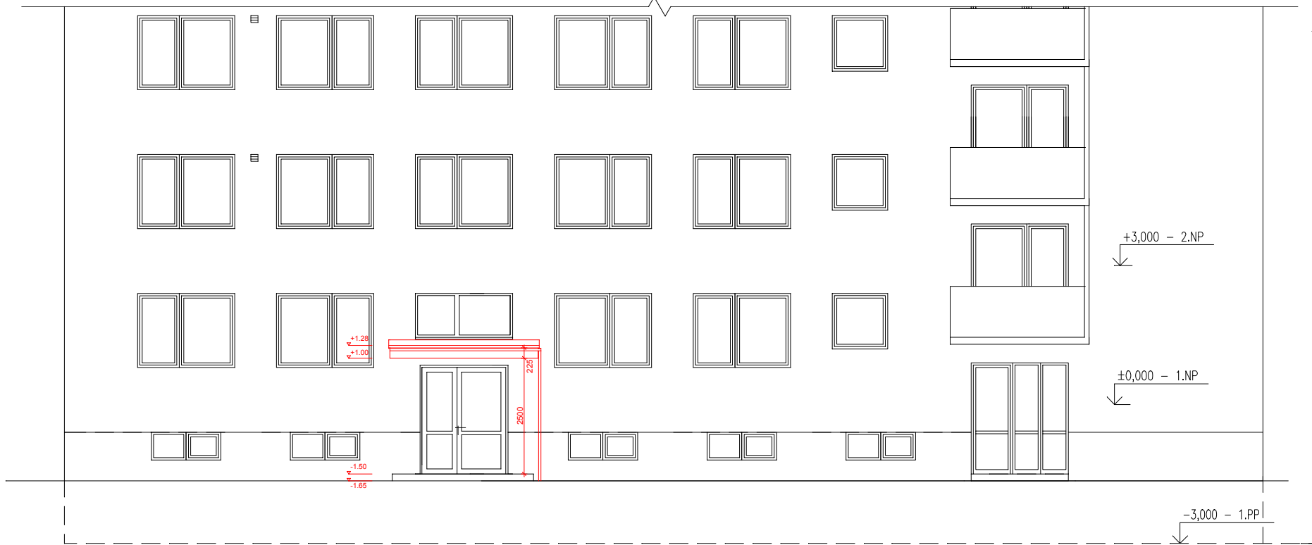
POHLED SEVEROZÁPADNÍ (OD KRYTÉHO BAZÉNU)
