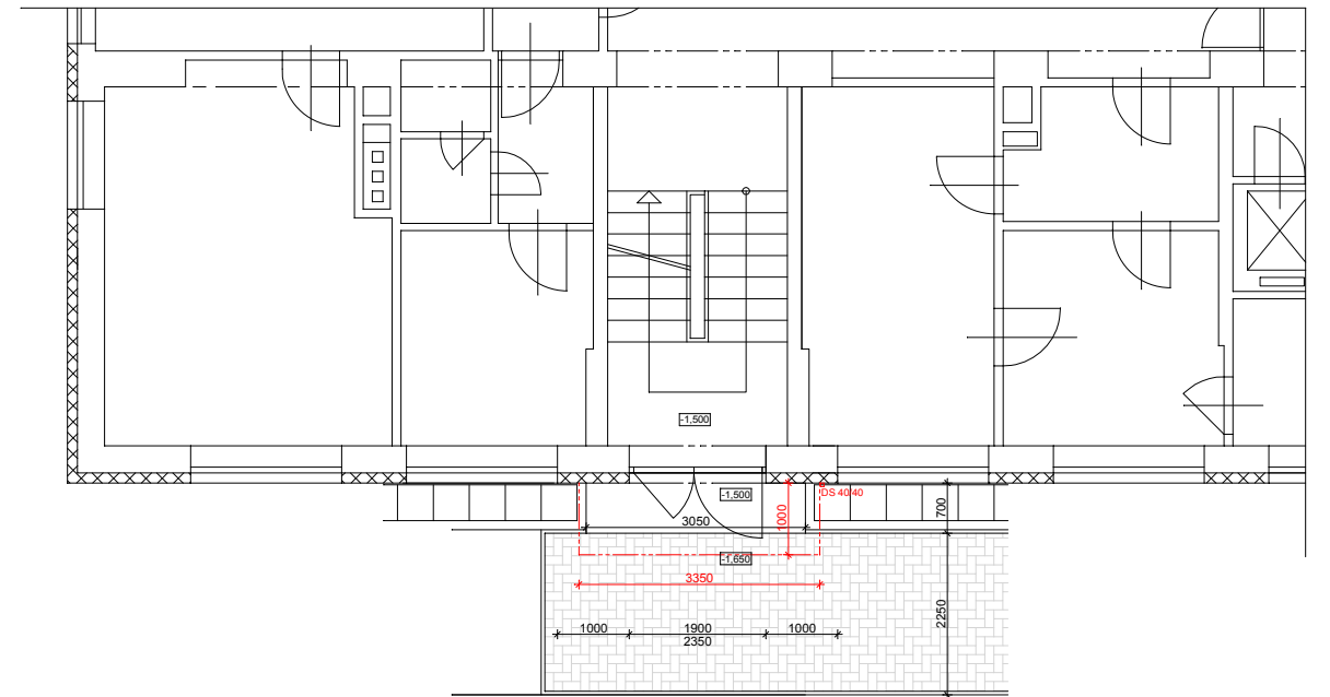
PŮDORYS 1.NP – objekt "E"
