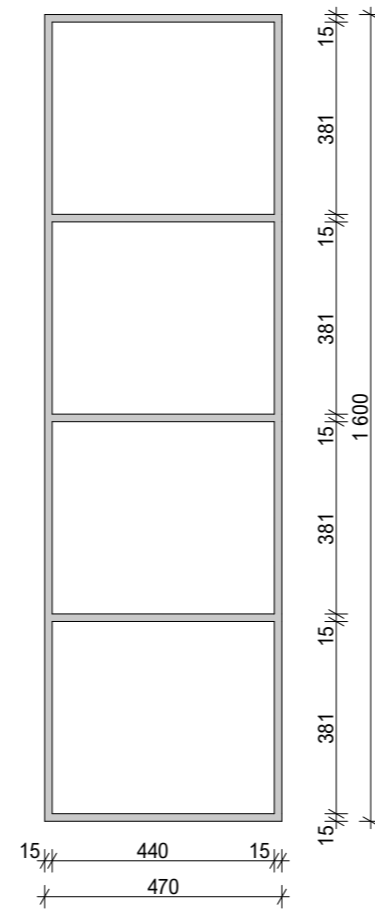
pohled boční
