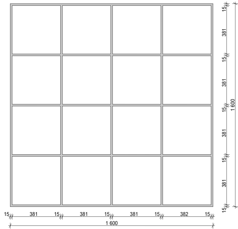
pohled čelní
