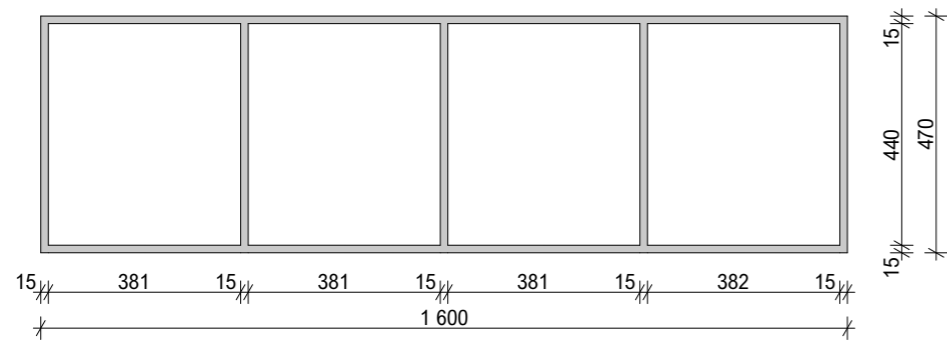
půdorys
