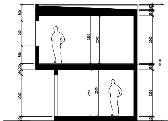
Řez
