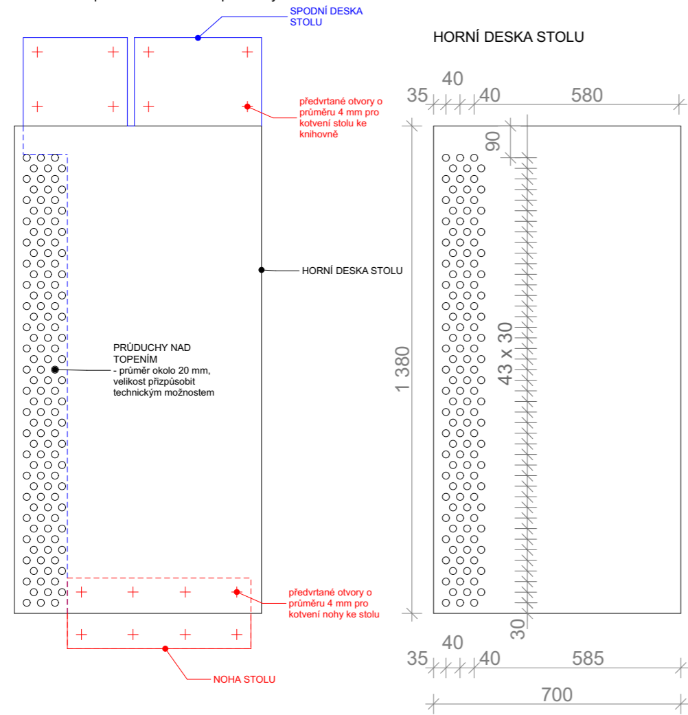
SCHÉMA STOLU - VAR 1 se spodní výztužnou deskou
