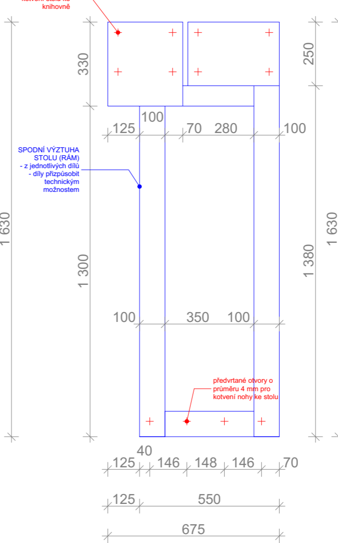
SCHÉMA STOLU - VAR 2 se spodní výztužným rámem z dílů
