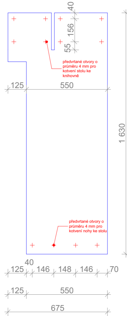
SCHÉMA STOLU - VAR 2 se spodní výztužným rámem z dílů
