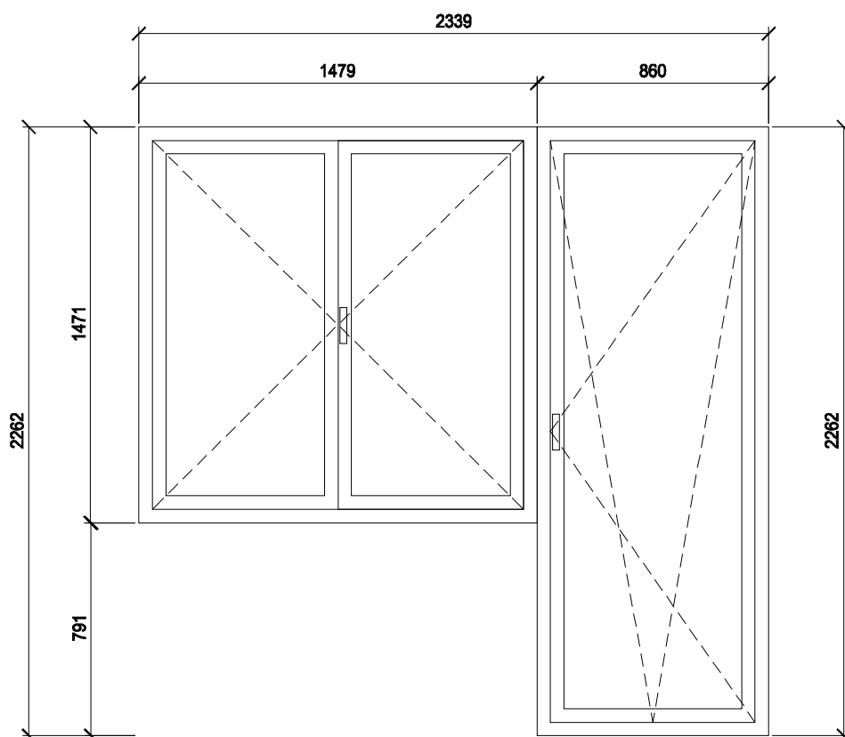
OKNO 5 _hala_vstup na terasu
