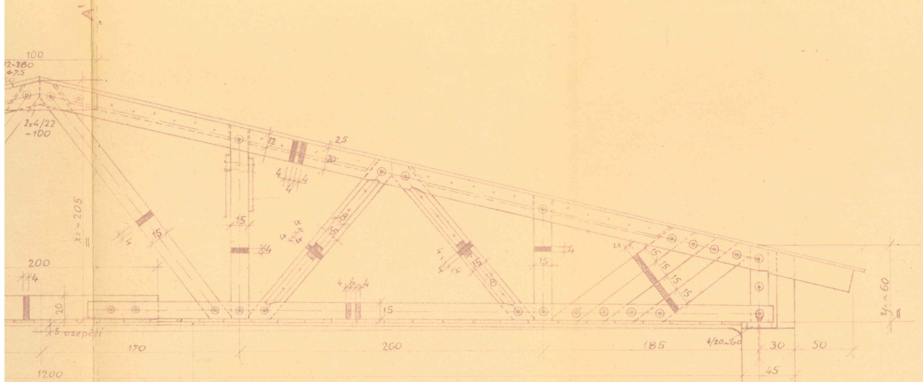
bednění 2cm rákos, omítka ČELNÝ NOSNÍK
