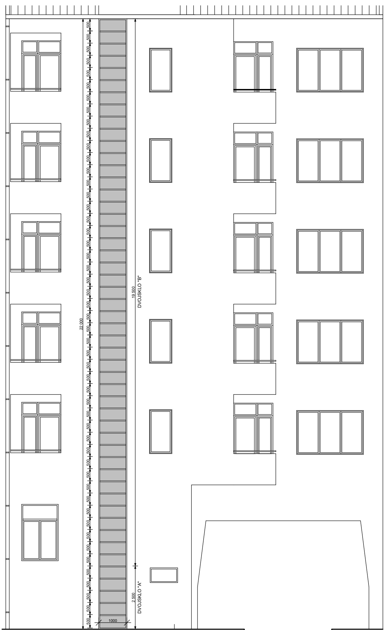
5 ks izolační dvojsklo "A" Float + Connex 39 ks izolační dvojsklo "B" 2x4 mm Float
