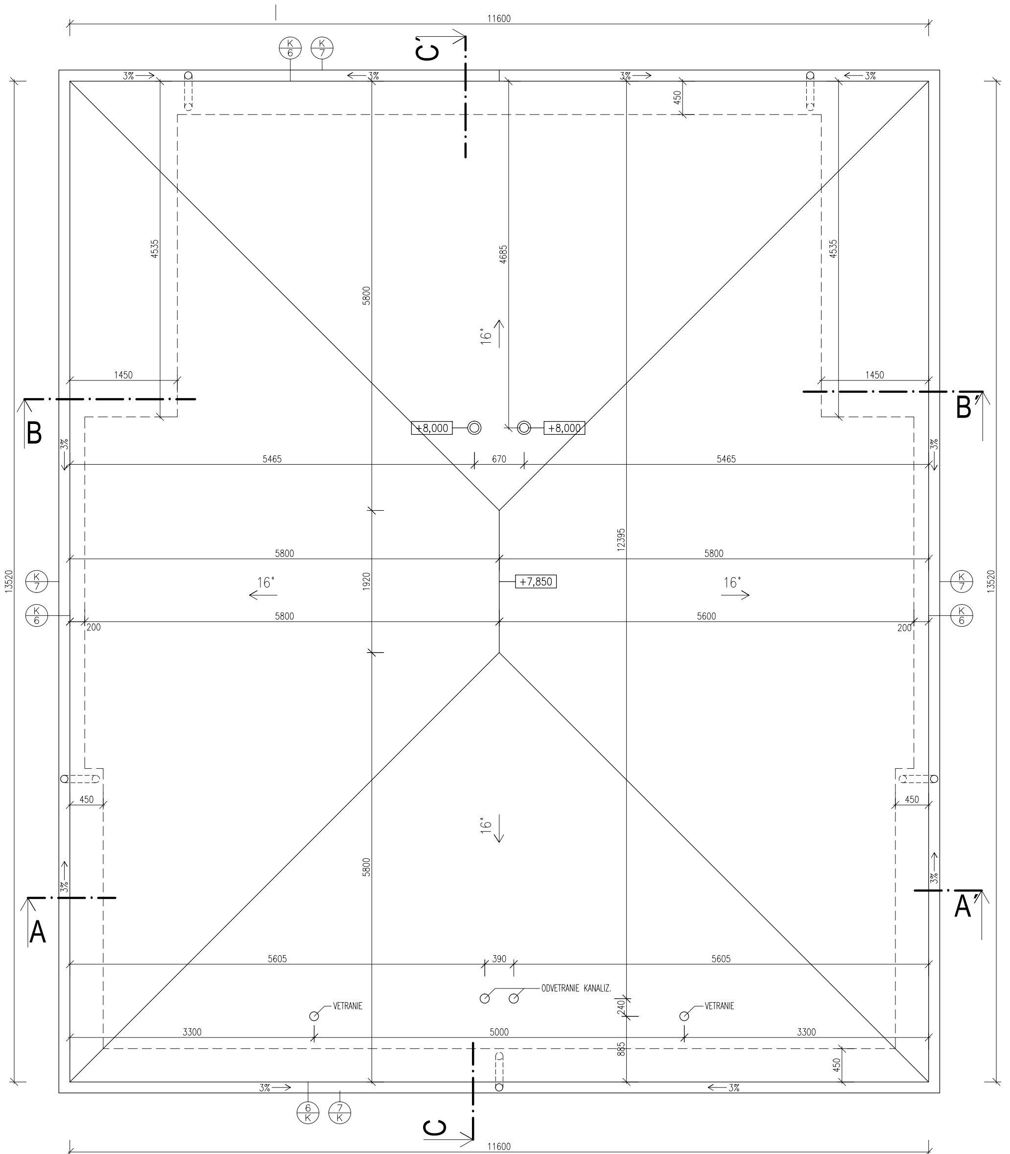
PÔDORYS STRECHY M 1:50
