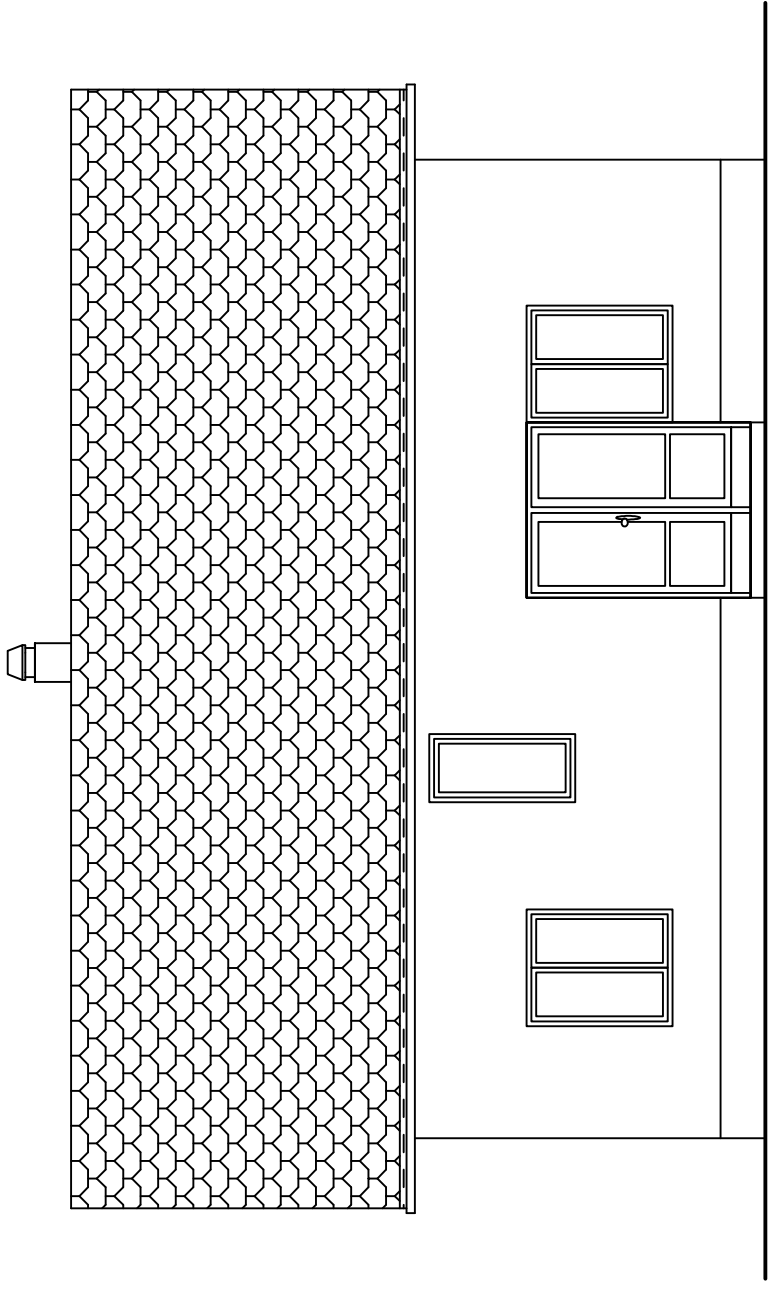
POHLED SEVEROVÝCHODNÍ
