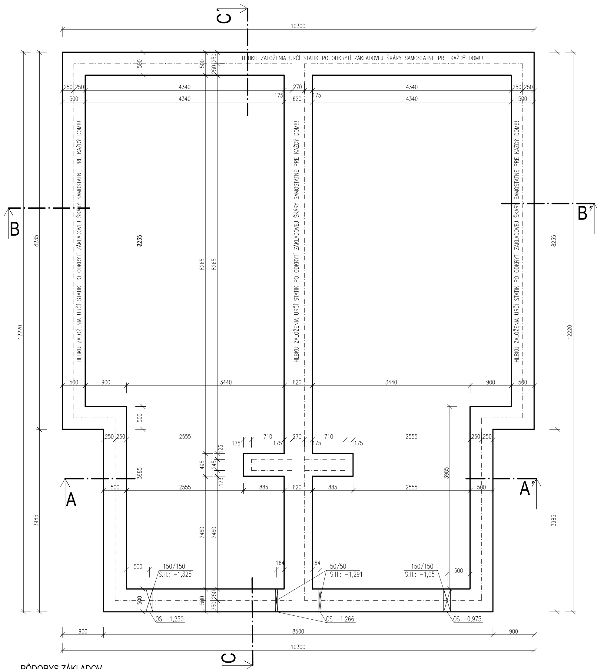
PÔDORYS ZÁKLADOV
