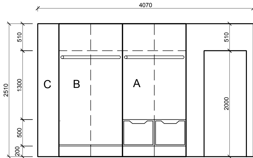
POHLED NA STĚNU 3
