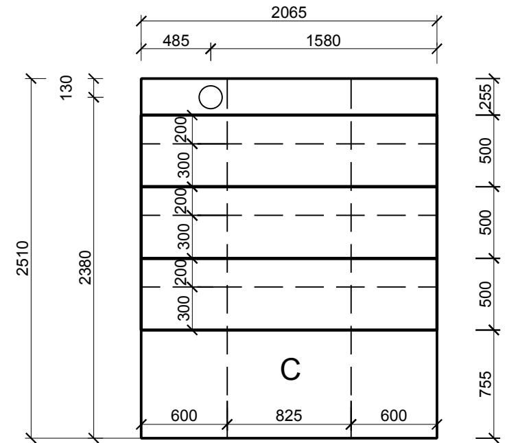
POHLED NA STĚNU 2
