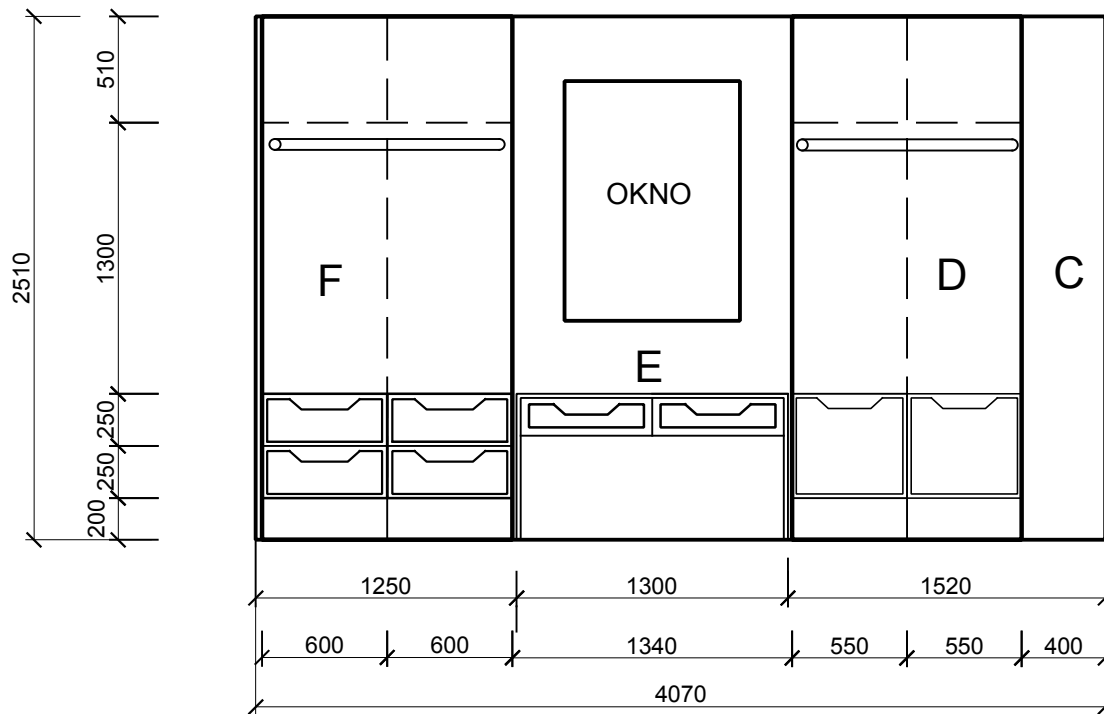
POHLED NA STĚNU 3
