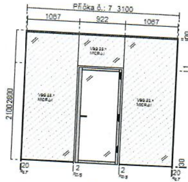
Příčka č.: 7
