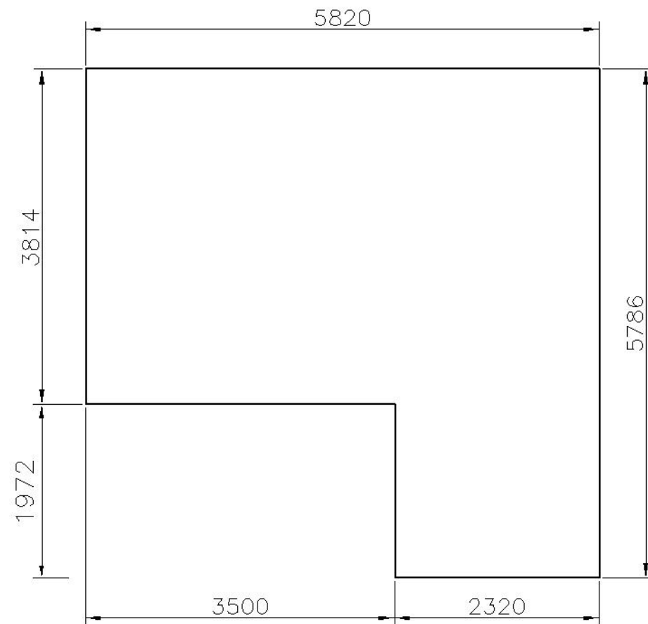
ROZMĚRY ZÁKLADOVÉ DESKY
