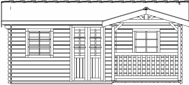
BOČNÍ POHLED LEVÝ
