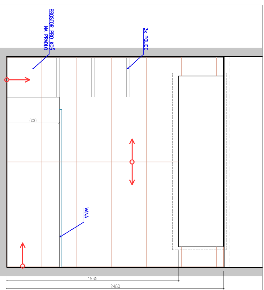
POHLED A
