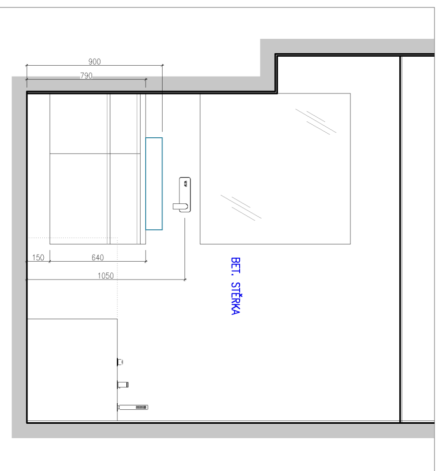
POHLED D
