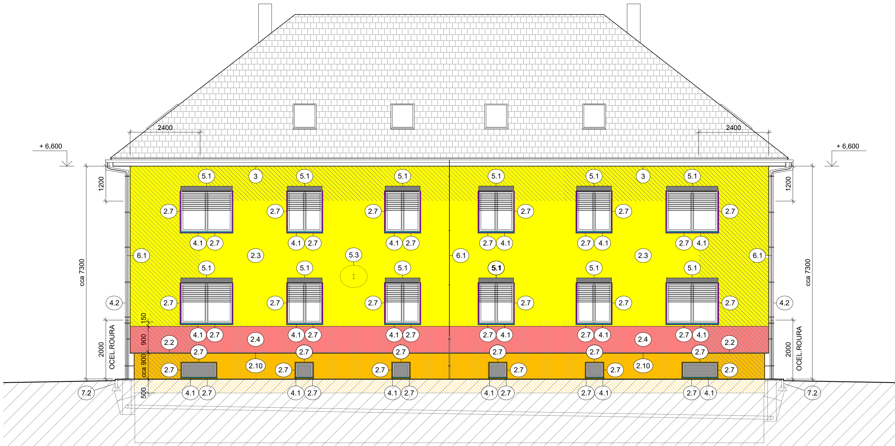
JIŽNÍ FASÁDA
