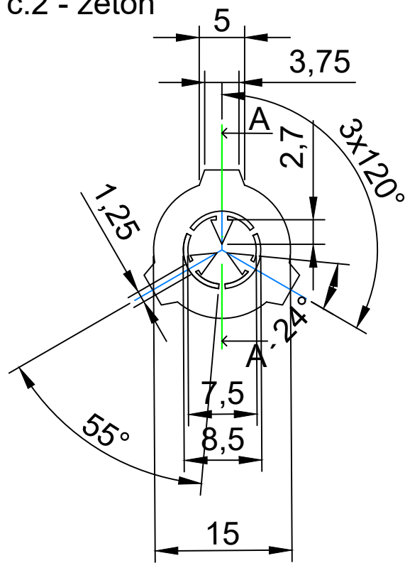
Řez A-A'
