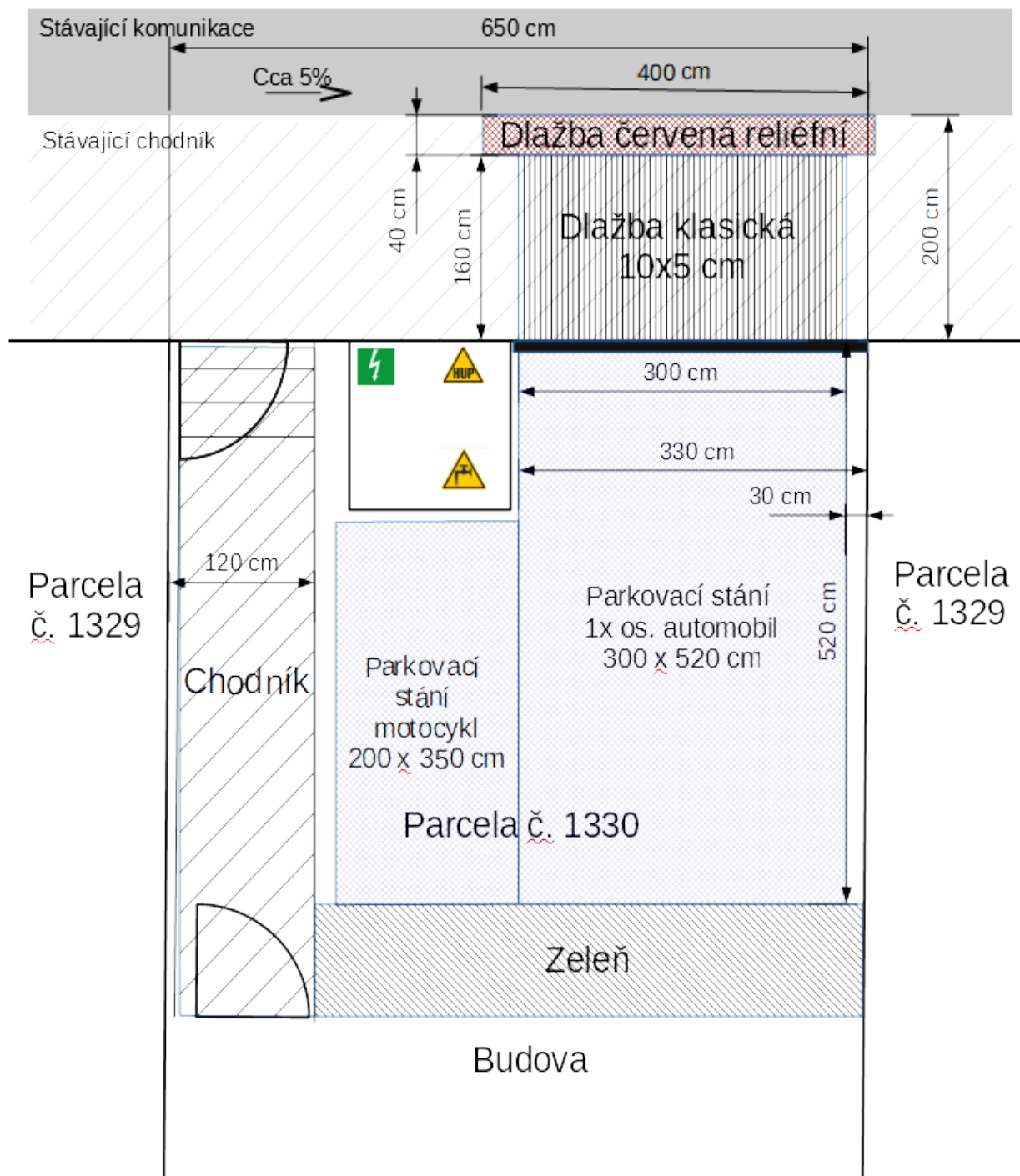
Schéma 2: Prostorové řešení sjezdu
