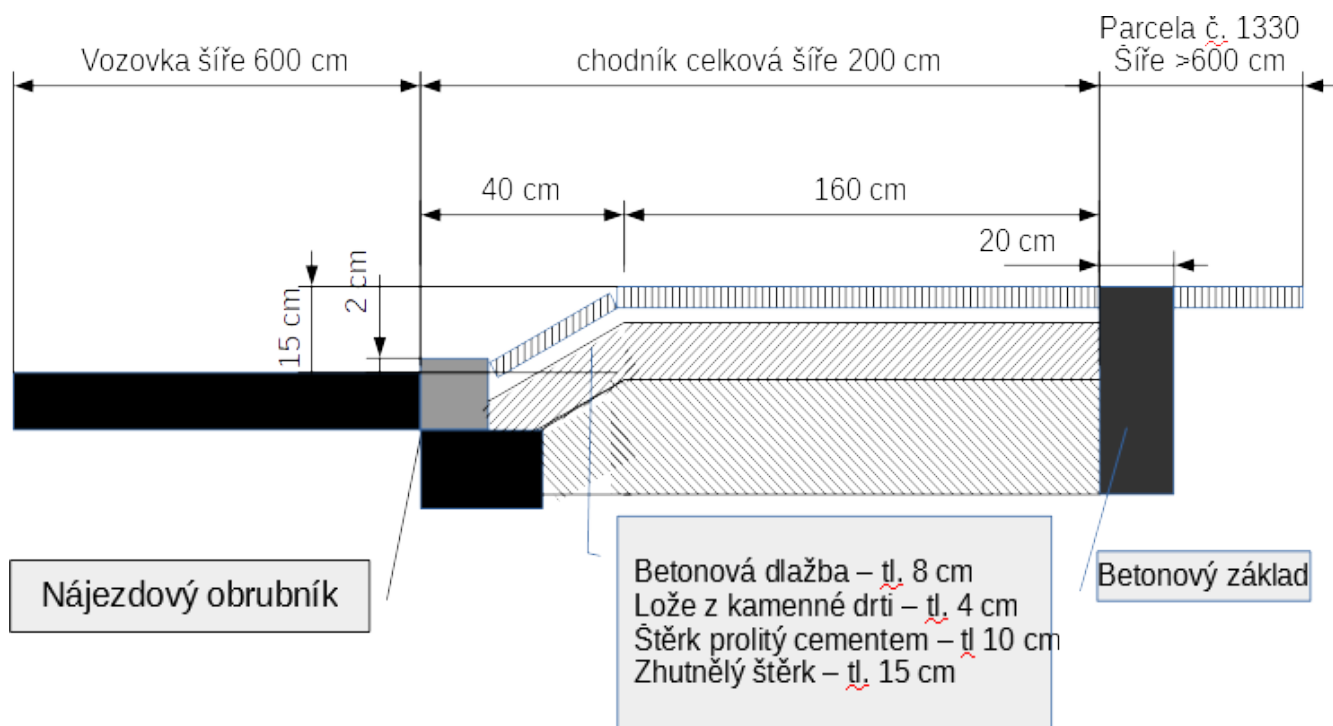
Schéma 1: Příčný řez
