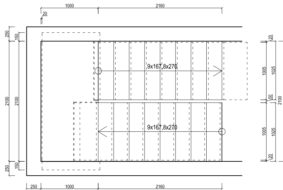
PŮDORYS 1NP
