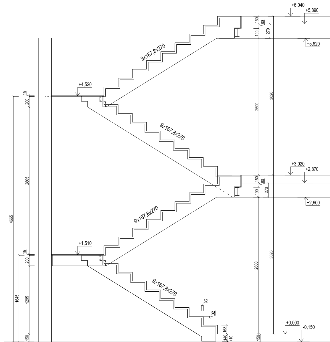
ŘEZ
