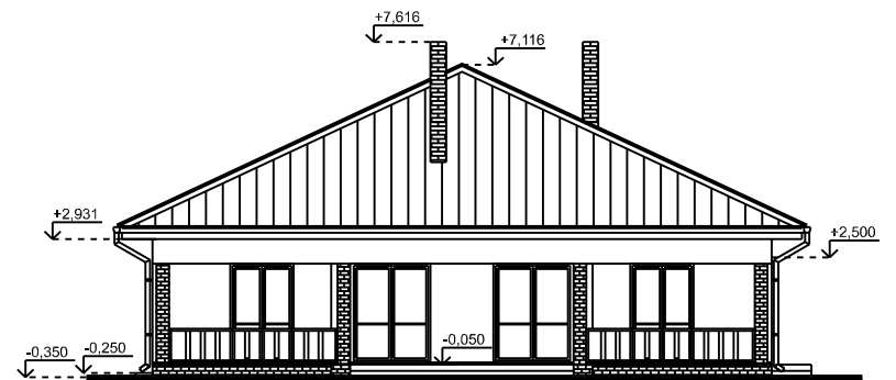
POHLAD ZÁPADNÝ
