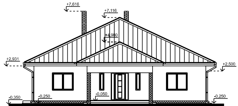
POHLAD VÝCHODNÝ
