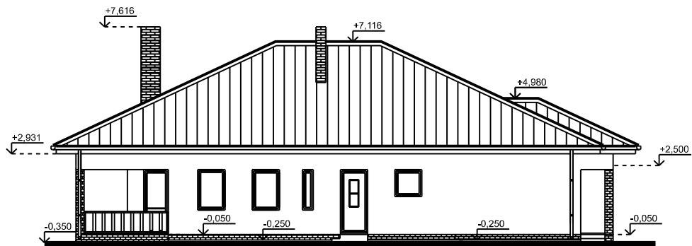
POHLAD JUŽNÝ
