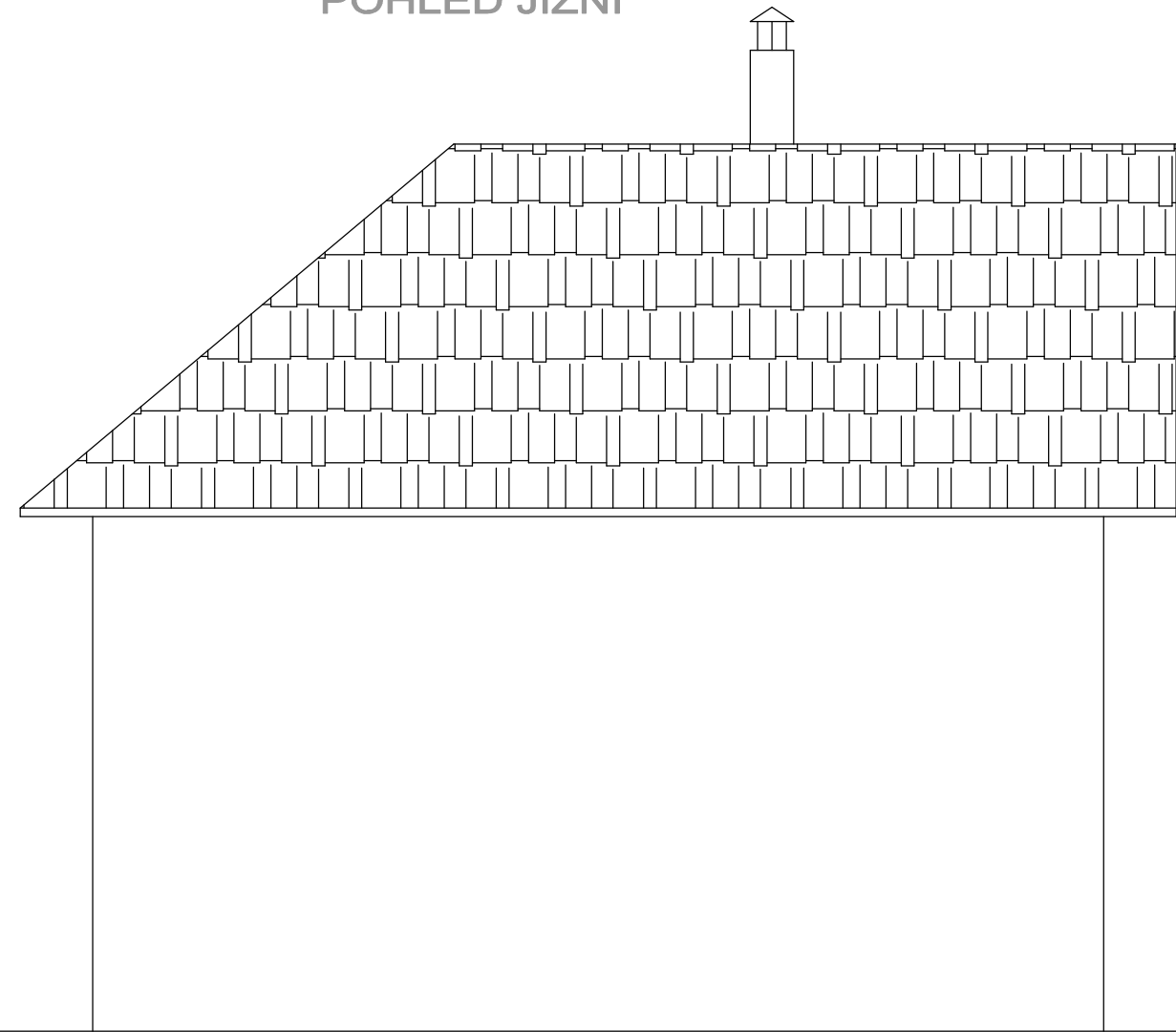
POHLED JIŽNÍ
