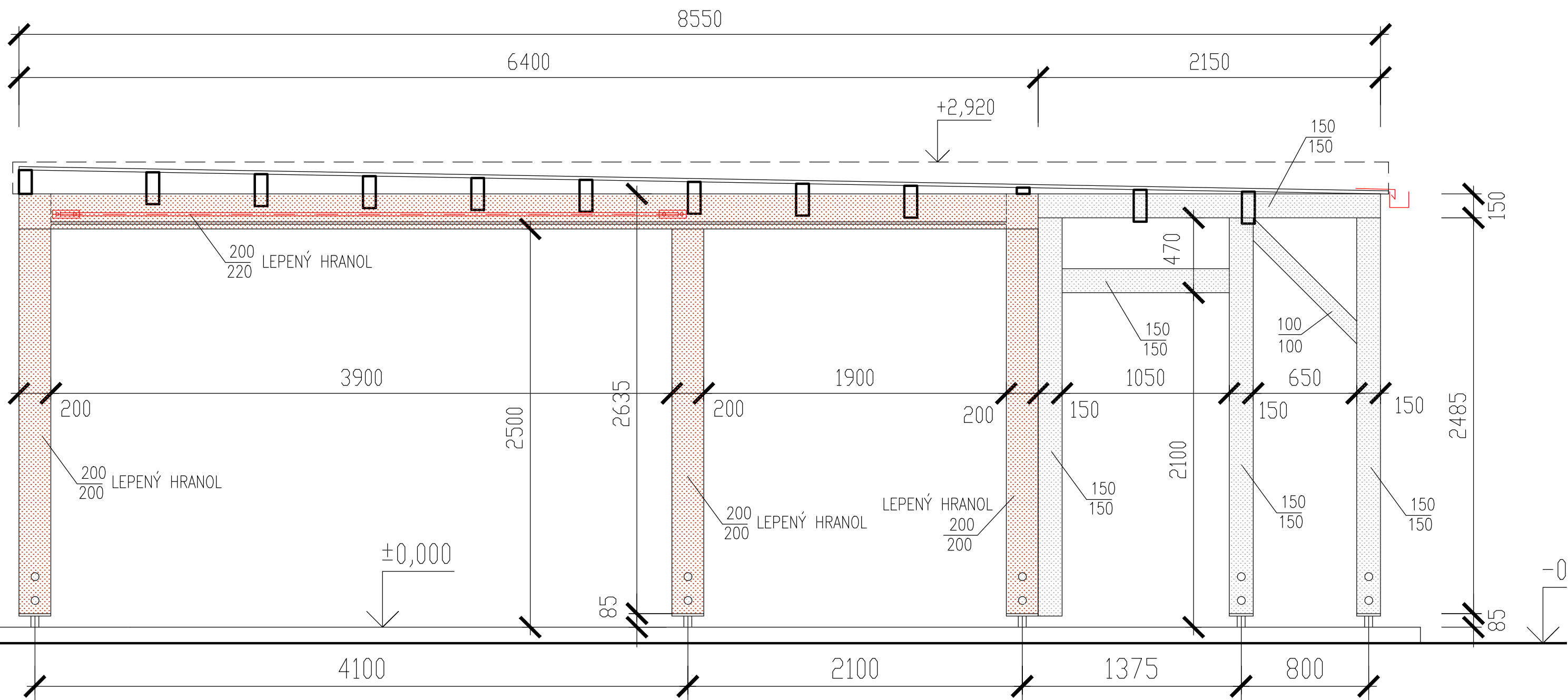
POHLAD BOČNÝ PRAVÝ
