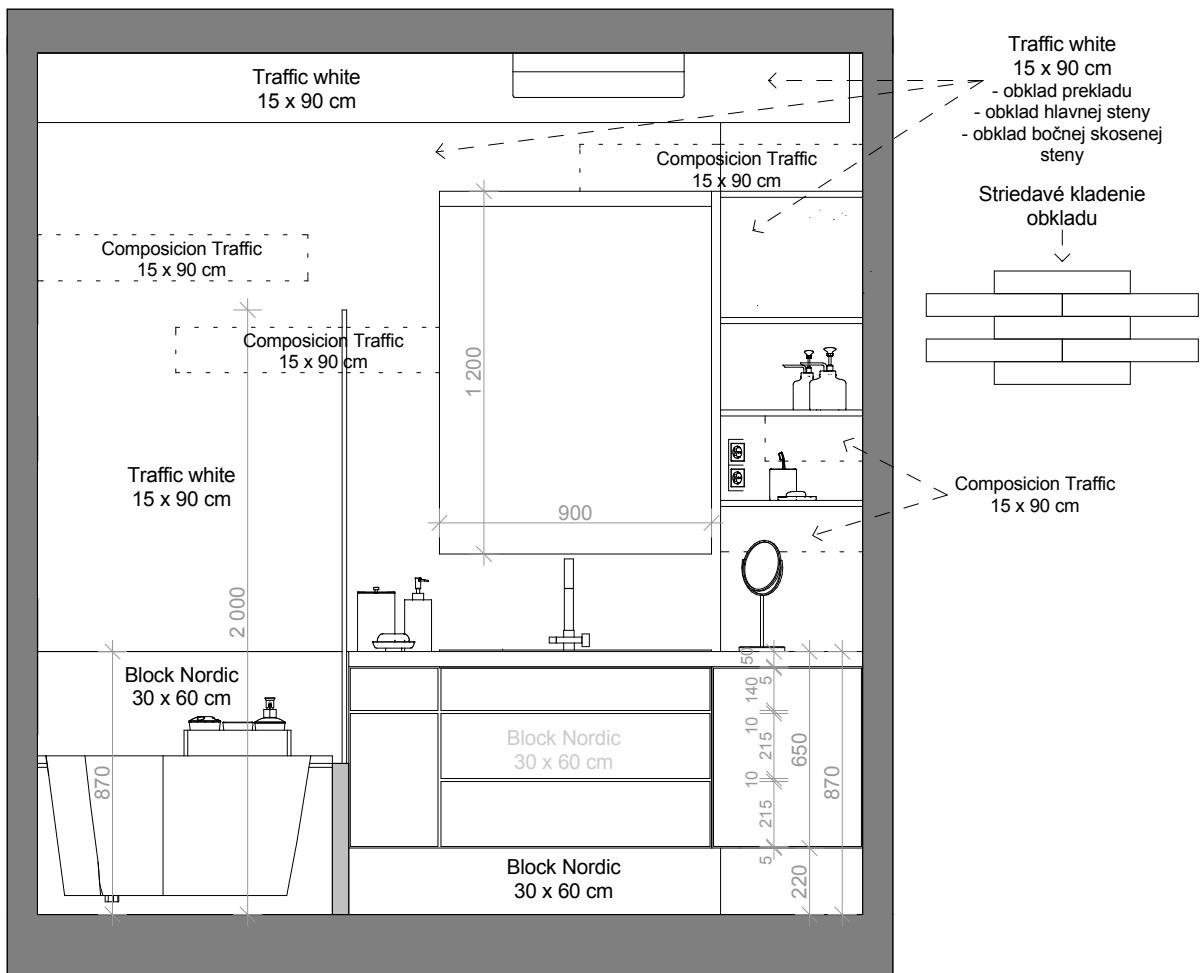
Kúpeľňa - pohľad A - čiarový
